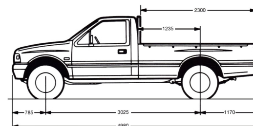
Normalkabine
