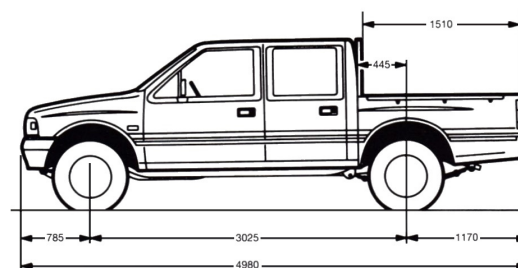
Mannschaftskabine
