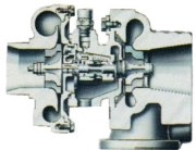
Mit dem Turbolader des Astra 1.7 TD ist beim Beschleunigen kein „Turboloch“ mehr zu spüren.
