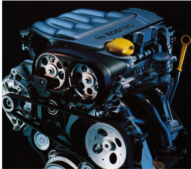
Optimierte Verbrennung: Gemischaufbereitung durch vier Ventile. Kurze Flammwege und effektivere Verbrennung durch zentral platzierte Zündkerze.
