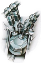
Optimierte Verbrennung: Gemischauflbereitung durch vier Ventile. Kurze Flammwege und effektivere Verbrennung durch zentral platzierte Zündkerze.
