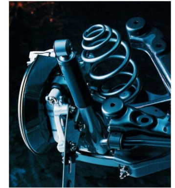
Hohe Quer- und Bremsstabilität. Die neue Vierlenker-Hinterachse in Leichtbauweise mit Radträger, Querlenker und Bremssätteln aus Aluminium.
