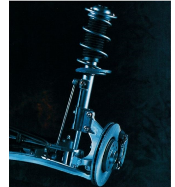
McPherson-Vorderachse mit hochfestem hydrogeformtem Fahrschemel. Querlenker und Achsschenkel aus Aluminium.
