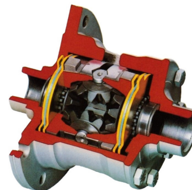
Sperrdifferential (Sonderausstattung). Sorgt unter allen Umständen für schlupffreies Anfahren und verbessert entscheidend das Kurvenverhalten.
