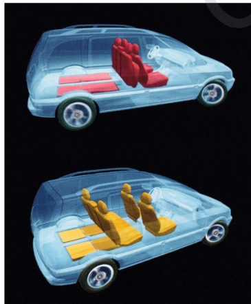
Noch mehr Variabilität dank optimiertem Flex7®-Sitzsystem – vom Zwei- zum Siebensitzer in wenigen Sekunden
