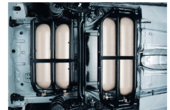
Die gesamte Tankanlage wird durch eine Unterbodenverkleidung geschützt
