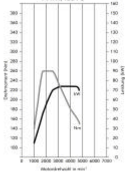
1.9 DTI ECOTEC® 74 kW/100 PS
