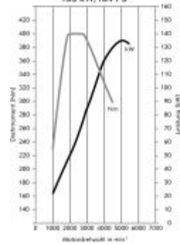
3.0 V6 CDTI ECOTEC® 135 kW/184 PS
